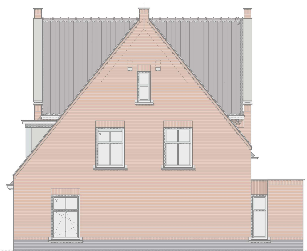
Rechter zijgevel
